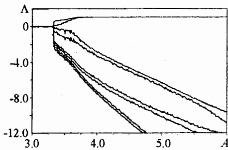
Рис. 5. Зависимость показателей Ляпунова от параметра глубины модуляции A при \omega_0 = 2\pi , T = 8 , \varepsilon = 0.6
