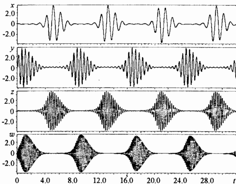
Рис. 2. Зависимости динамических переменных для составляющих систему четырех осцилляторов от времени при \omega_0 = 2\pi , T = 8 , A = 4.5 , \epsilon = 0.6
