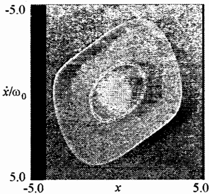
Рис. 4. Аттрактор в проекции на фазовую плоскость первого осциллятора. Белым цветом выделены точки, отвечающие максимуму значения бифуркационного параметра в первом осцилляторе, которые образуют портрет аттрактора в сечении Пуанкаре
