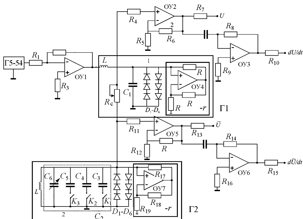
Рис. 4. Схема экспериментальной установки двух связанных автогенераторов под импульсным воздействием
