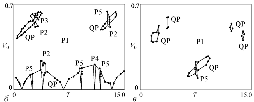
Рис. 6. Экспериментальная карта динамических режимов системы двух связанных автогенераторов ван дер Поля. a – без внешнего воздействия; b , в – с импульсным воздействием: b – в автономном режиме система демонстрирует режим захвата; в – в автономном режиме система демонстрирует гибель колебаний. Обозначения: P1, P2, и т.д. – режимы периода 1, 2 и т.д.; QP – квазипериодические режимы
