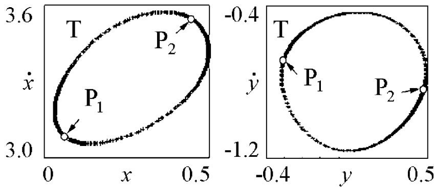
Рис. 2. Проекция стробоскопических сечений Пуанкаре на плоскости (x, \dot{x}) и (y, \dot{y}) : T – инвариантная кривая для квазипериодического режима, P_1, P_2 – 2-цикл, рождающийся из инвариантной кривой
