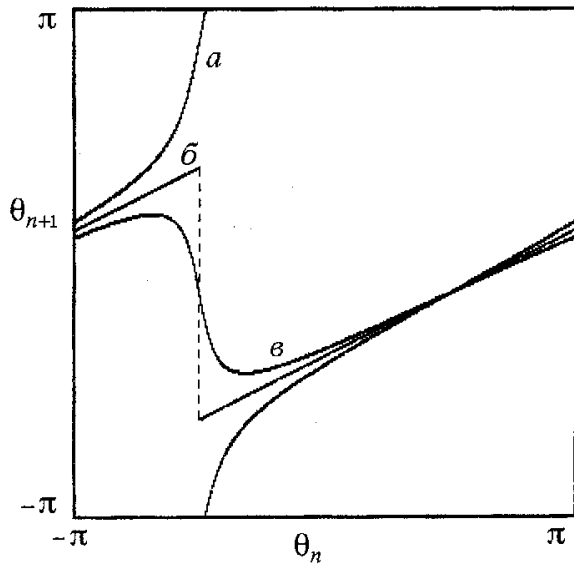
Рис. 2. Вид одномерного отображения (14) при различных C : а - 0.8, б - 1.0, в - 1.2
