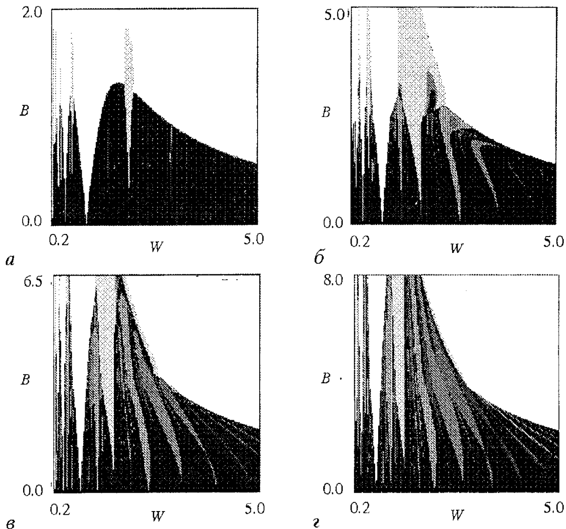
Рис. 10. Эволюция карт динамических режимов для генератора Ван дер Поля с импульсным воздействием при изменении параметра диссипации \lambda : a - 0.2; б - 1.2; в - 2.2; г - 3.2
