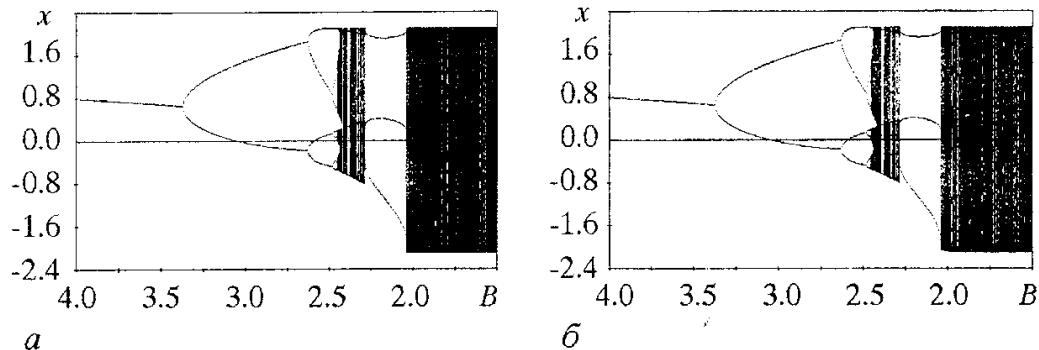
Рис. 9. Бифуркационные деревья одномерного отображения (а) и двумерного (б) при частоте воздействия W=0.725 и параметре \lambda=1.1 . Используются переменные, характерные для двумерного отображения
