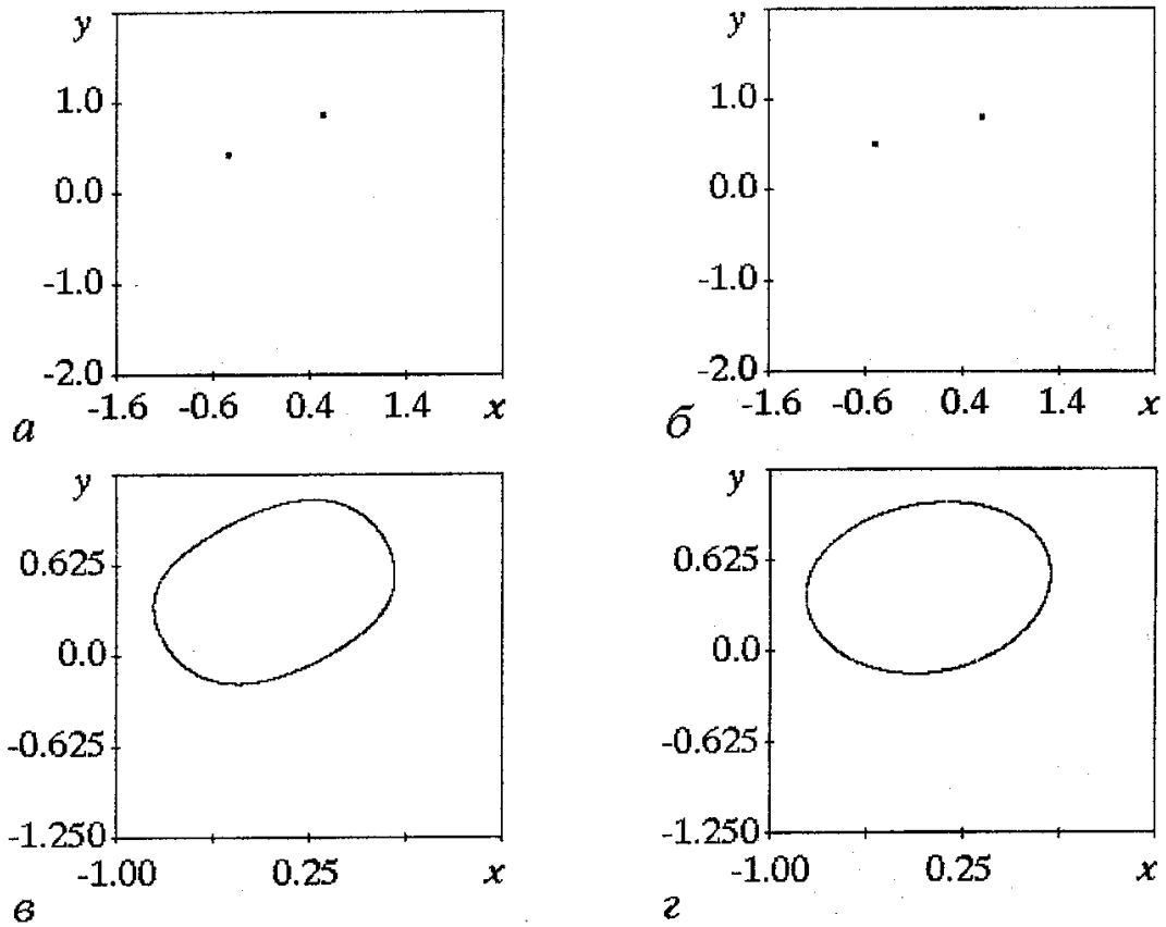
Рис. 11. Сечения Пуанкаре для генератора Ван дер Поля (а, в) и портреты аттракторов двумерного отображения (15) (б, г) при W=2.05 ; B=1.3 (а, в); B=0.8 (б, г). Значение параметра диссипации \lambda=0.2
