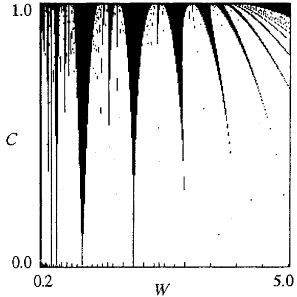
Рис. 5. Картина языков синхронизации для одномерного отображения (14) на плоскости амплитуды воздействия C , частота W в области C_1
