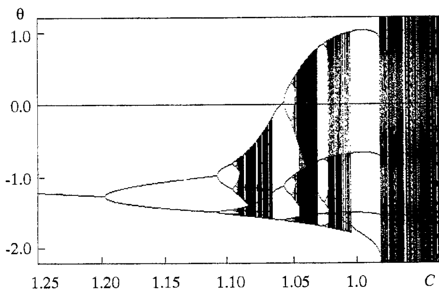
Рис. 4. Бифуркационное дерево для одномерного отображения (14) при уменьшении амплитуды C . Частота воздействия W=3.2
