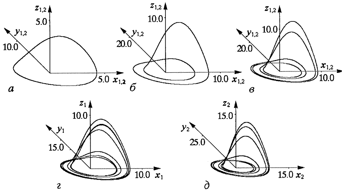
Рис. 14. Фазовые портреты для связанных осцилляторов Ресслера (19) при тех же значениях параметров, что и на рис. 13. Представлены аттракторы периода 1 (а), 2 (б), 4 (в) и 6 (з, д). Заметим, что при равных значениях параметров c_1 и c_2 , значения переменных в парциальных системах совпадают (а-в). В случае c_1 \neq c_2 (з, д), когда могут реализоваться феномены комплексной аналитической динамики такие, например, как утроения периода, значения динамических переменных парциальных систем не совпадают
