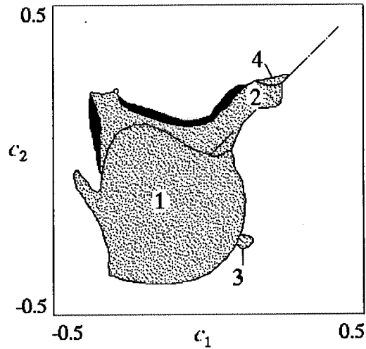
Рис. 10. Плоскость параметров (c_1, c_2) для связанных осцилляторов Ресслера (17) при \epsilon=0.5 , a=0.2 , b=0.2
