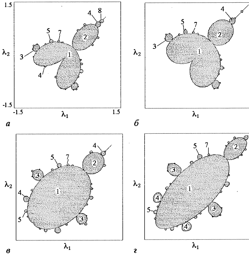
Рис. 4. Множества Мандельброта для связанных отображений Эно (9) при следующих значениях параметра d : -0.5 (а); -0.3 (б); 0.3 (в); 0.5 (г). Параметр связи \varepsilon=0.5
