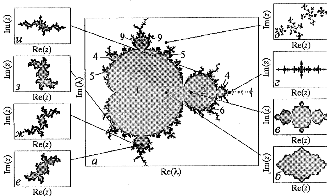
Рис. 1. Множество Манделъброта ( a ) и множества Жюлиа для квадратичного комплексного отображения при различных значениях параметра \lambda : 0.5 ( б ), 0.8 ( в ), 1.42 ( з ), 0.5+0.7i ( д ), 0.123-0.745i ( е ), 0.0315-0.7908i ( ж ), -0.282+0.530i ( з ), 1.16+0.25i ( и ). Серым цветом на рисунках обозначены области, которым соответствует существование периодической динамики (периоды указаны цифрами); черным цветом обозначены точки, в которых реализуется ограниченная в фазовом пространстве хаотическая динамика; белый цвет означает убегание траекторий на бесконечность
