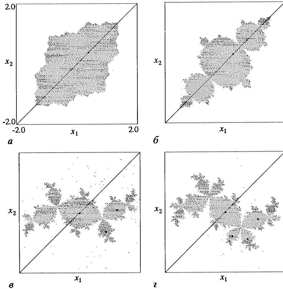
Рис. 3. Фазовые плоскости (x_1, x_2) для связанных логистических отображений при значении параметра связи \epsilon = 0.5 для следующих значений параметров \lambda_1 и \lambda_2 : \lambda_1 = \lambda_2 = 0.5 (а); \lambda_1 = \lambda_2 = 0.8 (б); \lambda_1 = 0.868, \lambda_2 = 0.622 (в); \lambda_1 = 0.248, \lambda_2 = 0.812 (г). Точками обозначены аттракторы, а серым цветом - их бассейны притяжения. Приведены рисунки для неподвижной точки (а) и циклов периода 2 (б), 3 (в), 4 (г)
