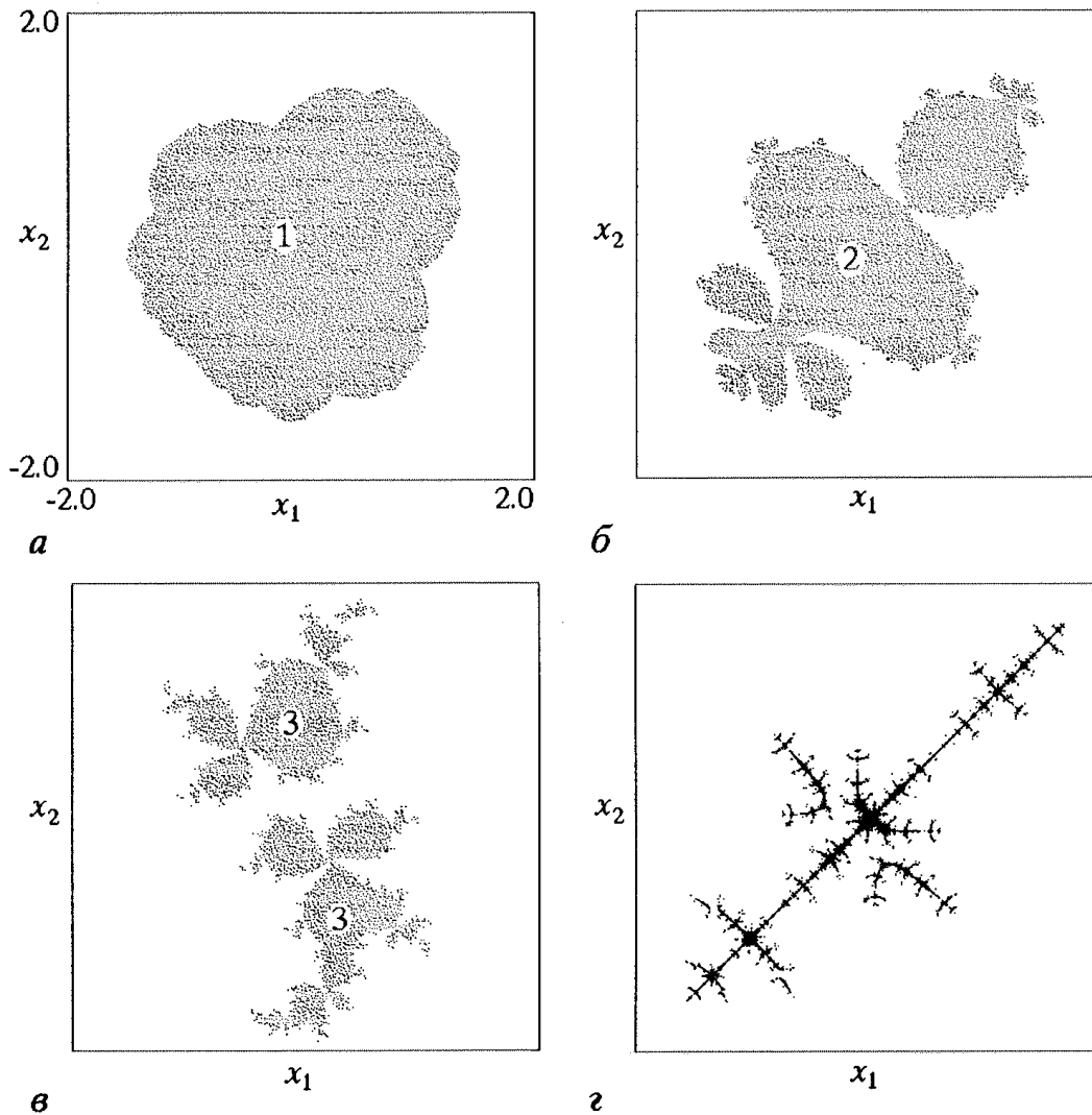
Рис. 5. Множества Жюлиа для связанных отображений Эно при d=-0.3 для следующих значений параметров \lambda_1 и \lambda_2 : \lambda_1=\lambda_2=0.1 (а); \lambda_1=\lambda_2=0.5 (б); \lambda_1=-0.8, \lambda_2=0.5 (в); \lambda_1=\lambda_2=1.05 (г)
