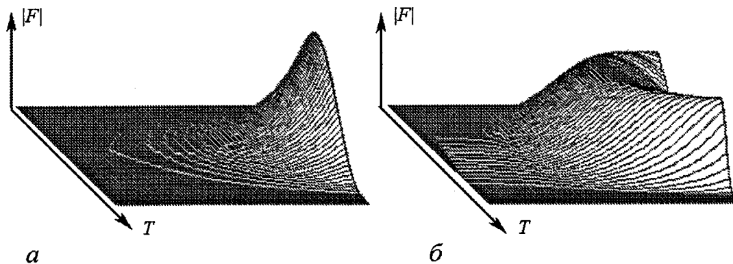
Рис. 4. Изменение во времени распределения амплитуды поля по длине системы; A=0.5 , \alpha=0.05 , L=6.0 . a - Линейная теория, максимальное значение |F| \approx 51.0 ; б - нелинейная теория, |F| \approx 3.0
