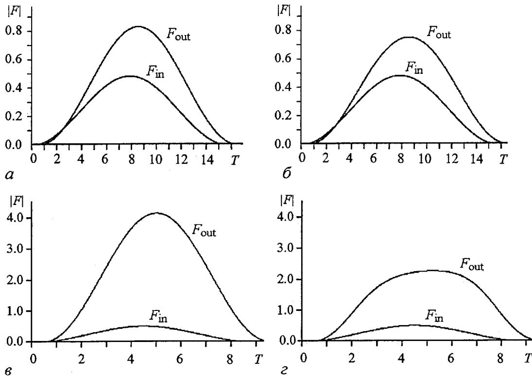
Рис. 3. Зависимости амплитуд входных F_{in} и выходных F_{out} сигналов от времени; A=1.0 , \alpha=0.1 . a ( L=2 ) и б ( L=3.5 ) - линейная теория; в ( L=2 ) и г ( L=3.5 ) - нелинейная теория
