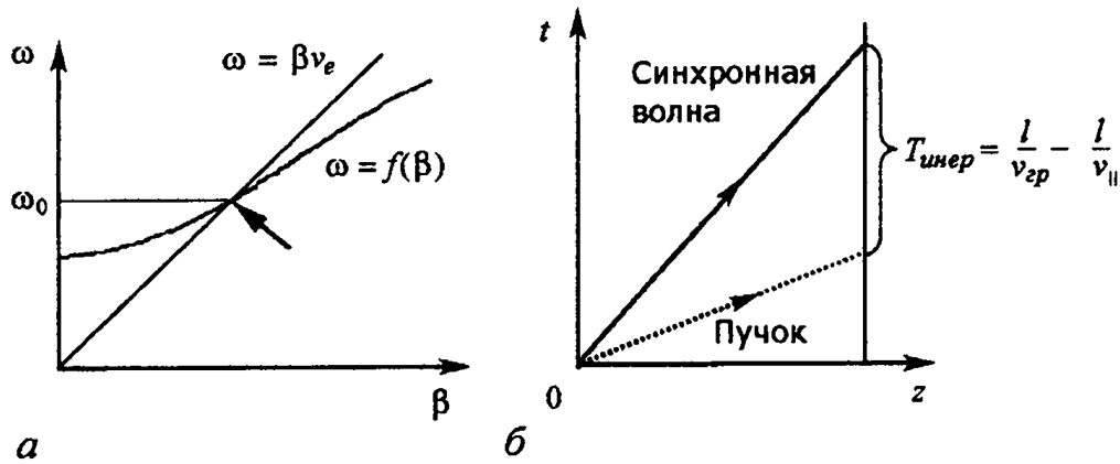
Рис. 1. a - Дисперсионные характеристики электронного пучка и электромагнитной волны. б - Пространственно-временная диаграмма; наклон линии синхронной волны отвечает групповой скорости
