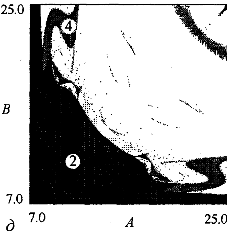
Рис. 7. Карты динамических режимов системы связанных осцилляторов Дuffинга (3) на плоскости (A, B) при различных значениях параметра связи: a - 0.2, б - 0.3, в - 0.5, г - 0.7, д - 0.8, e - 1.0 . При построении карт рассматривались периоды, кратные двум. Параметры \gamma=0.2 и \omega=1.46 . Цифрами отмечены области существования циклов различных периодов
