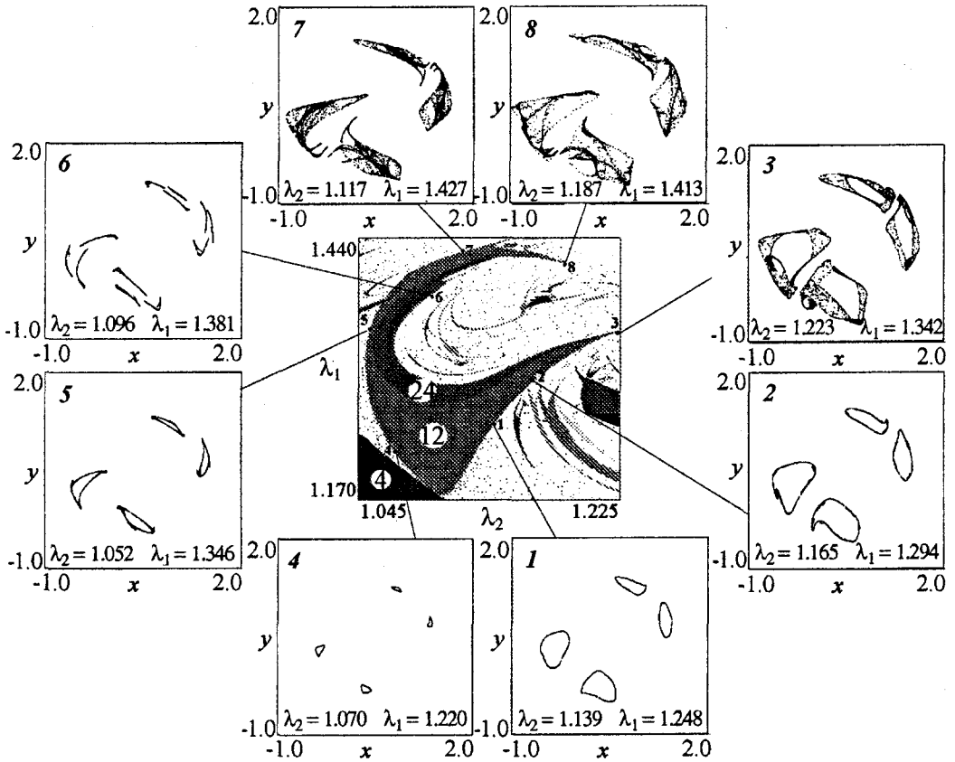
Рис. 4. Фазовые портреты аттракторов системы (2) в различных точках плоскости параметров (\lambda_2, \lambda_1) для значения параметра связи \epsilon=0.4 . В центре представлена карта динамических режимов для \epsilon=0.4 . Точные координаты (\lambda_2, \lambda_1) каждой выбранной точки на карте указаны в соответствующем фрагменте
