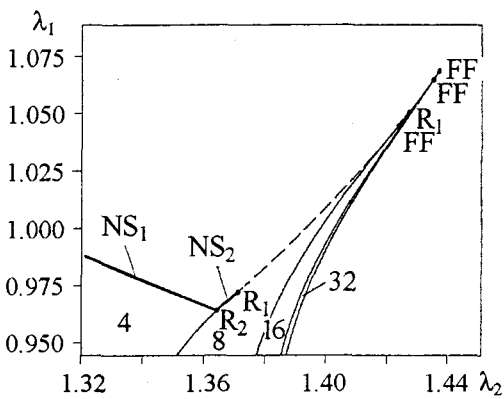
Рис. 6. Увеличенный фрагмент рис. 5, б. Цифрами отмечены области существования циклов периодов 4, 8, 16 и 32; сплошные линии соответствуют линиям бифуркаций удвоения периода, прерывистые - линиям жесткого перехода, жирные - линиям бифуркаций Неймарка - Сакера NS
