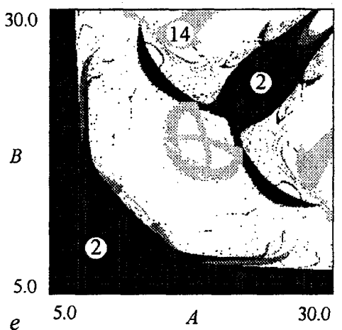
Рис. 7. Карты динамических режимов системы связанных осцилляторов Дuffинга (3) на плоскости (A, B) при различных значениях параметра связи: a - 0.2, б - 0.3, в - 0.5, г - 0.7, д - 0.8, e - 1.0 . При построении карт рассматривались периоды, кратные двум. Параметры \gamma=0.2 и \omega=1.46 . Цифрами отмечены области существования циклов различных периодов
