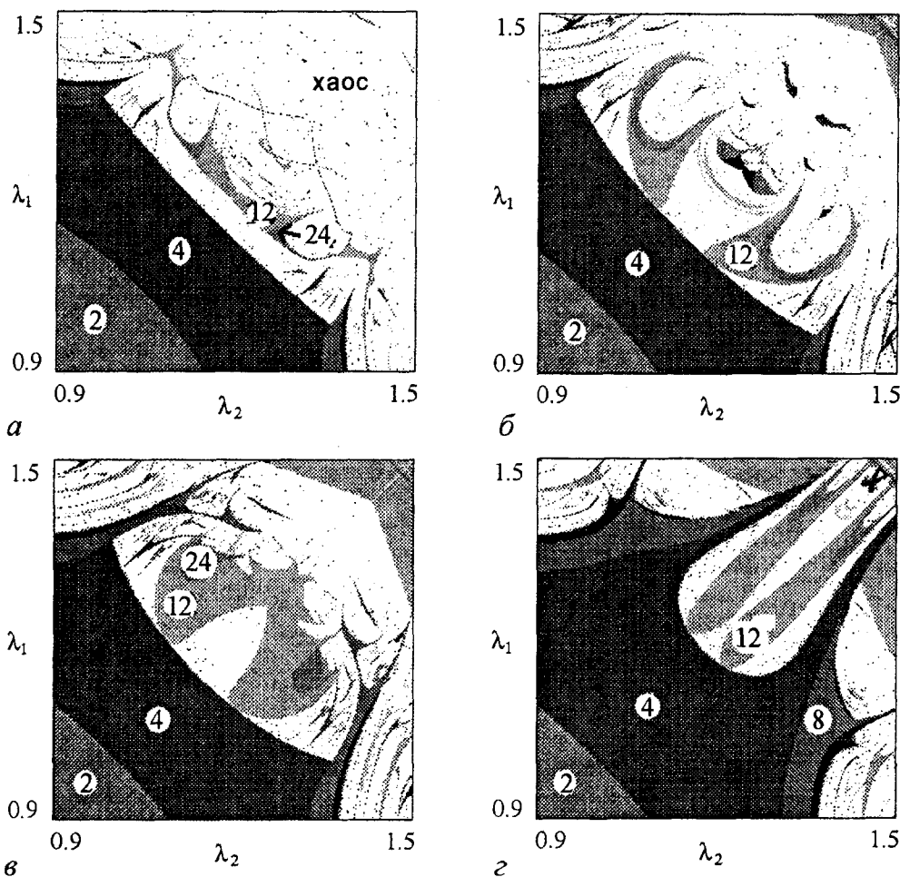
Рис. 3. Трансформация языков синхронизации системы (2) на плоскости (\lambda_2, \lambda_1) в диапазоне параметра диссипации \epsilon от 0.3 до 0.49: а - 0.3, б - 0.4, в - 0.44, г - 0.49
