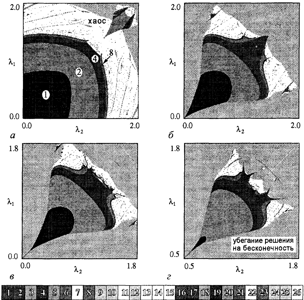
Рис. 2. Карты динамических режимов системы неидентичных связанных логистических отображений (2) на плоскости (\lambda_2, \lambda_1) при различных значениях параметра связи: а - 0.2, б - 0.5, в - 0.6, г - 0.9
